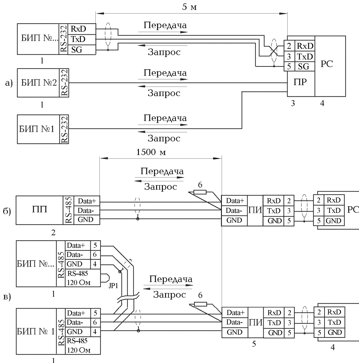
Схема подключения ПЭВМ (IBM PC) к расходомерам-счетчикам ИРВИС-РС4-Ультра с использованием интерфейса RS232/485
